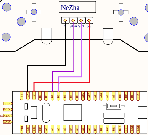
stm32最小系统板
